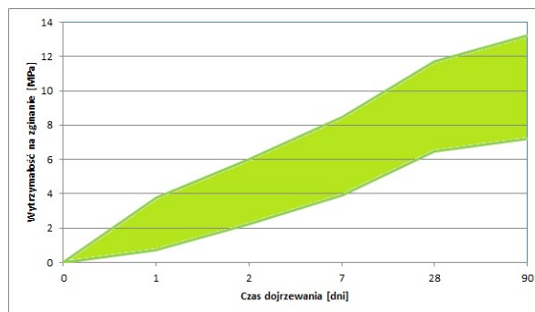
Rys.2. Wykres wytrzymałości na rozciąganie przy zginaniu produktu INIEKTON, w zależności od czasu dojrzewania (w temperaturze 20°C).
