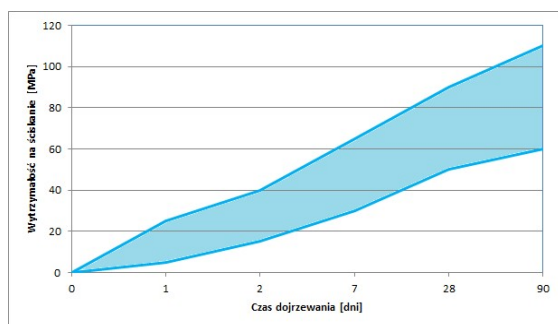
Rys.1. Wykres wytrzymałości na ściskanie produktu INIEKTON, w zależności od czasu dojrzewania (w temperaturze 20°C).
